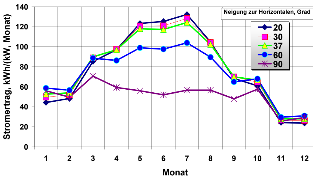
Abb. 15a: Stromertrag einer 3-kW PV-Anlage: Simulation, in Abhängigkeit von Orientierung und Ausrichtung des Solargenerators
