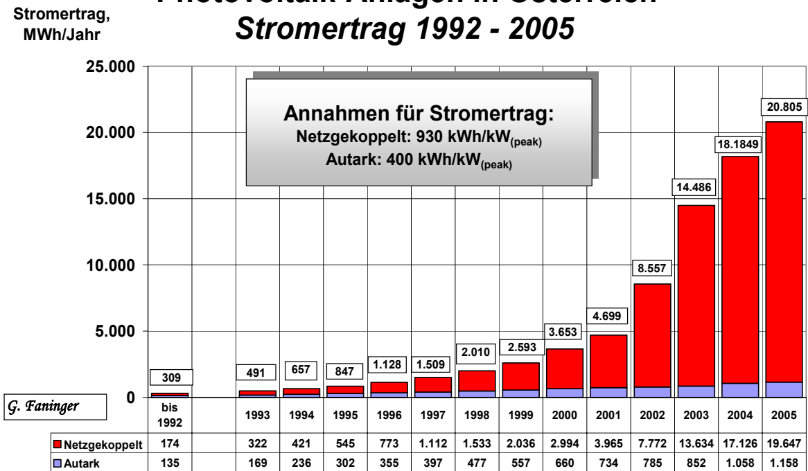
Abb. 18a: Stromertrag von Photovoltaikanlagen in Österreich: 1992 – 2005 Optimale Voraussetzungen
