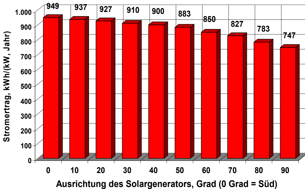
Abb. 15c: Stromertrag einer 3-kW PV-Anlage: Simulation, in Abhängigkeit von der Ausrichtung des Solargenerators
