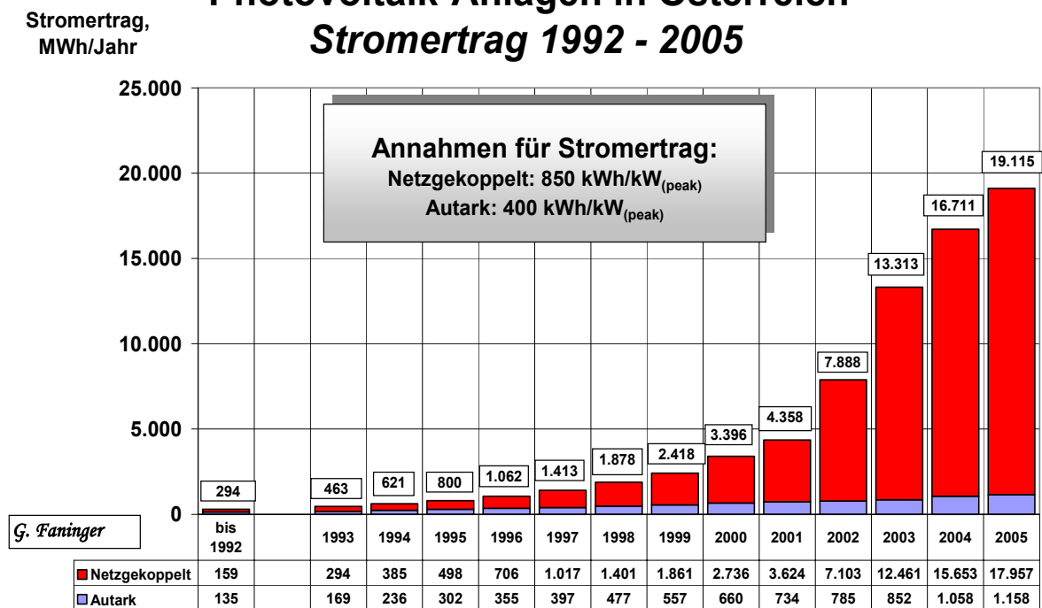
Abb. 18b: Stromertrag von Photovoltaikanlagen in Österreich: 1992 – 2005 Durchschnittliche Voraussetzungen
