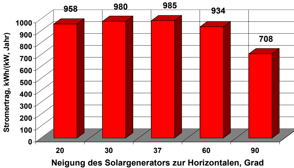
Abb. 15b: Stromertrag einer 3-kW PV-Anlage: Simulation, in Abhängigkeit von der Neigung des Solargenerators
